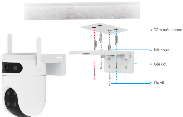
Hình 1 Gắn trần
