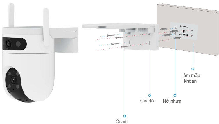
Hình 2 Gắn tường
