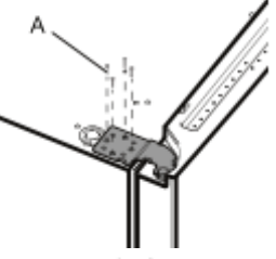
A. Vít ổ cắm 5mm
