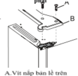
A. Vít nắp bản lề trên cùng B. Vít ổ cắm 5mm
