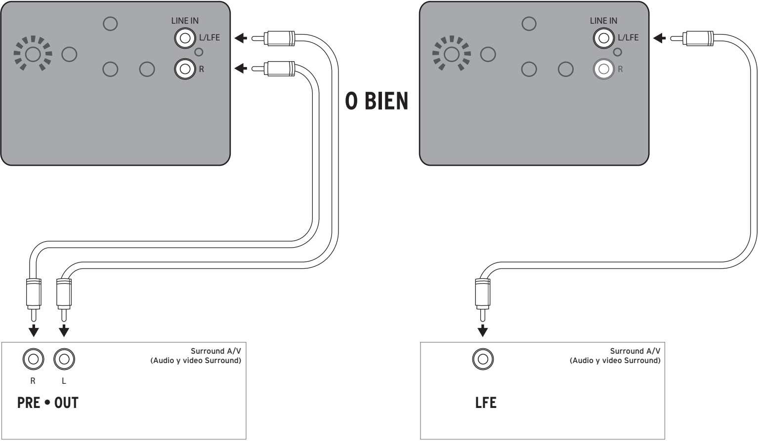
FIGURA 2 CABLEADO DE LOS SUBWOOFERS R-100SW Y R-120SW
