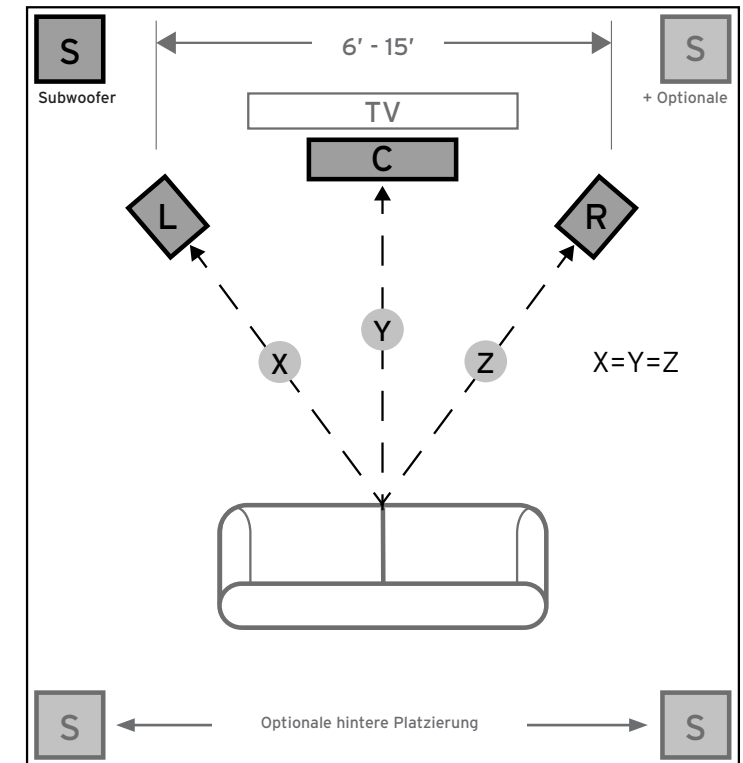
ABBILDUNG 1 LAUTSPRECHERPLATZIERUNG IM HÖRBEREICH
